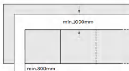
图3 后出线柜体距离墙面的距离
