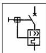
断路器（带热过载保护）
