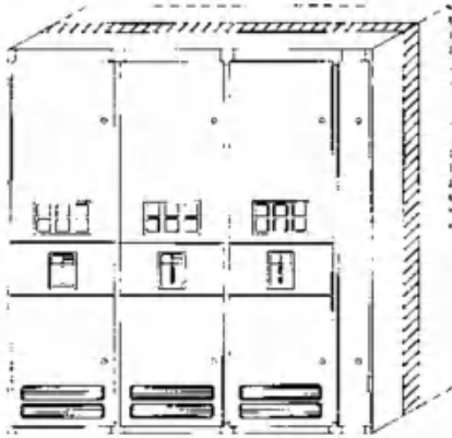
带有空气断路器的装置小室，母线小室、母线连接小室的开关柜
