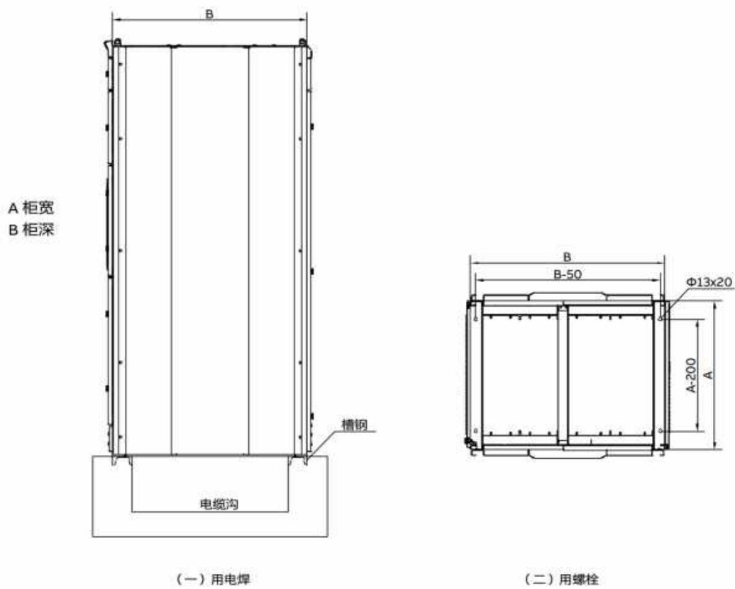
图5 安装基础图
